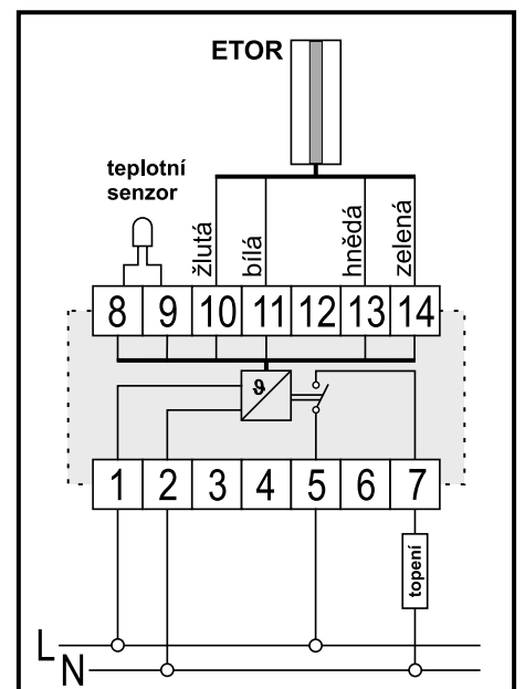
schéma zapojení ETR2 s čidly ETOR a ST pro ochranu okapů
