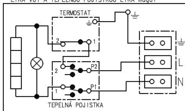
SCHEMA ELEKTRICKÉHO ZAPOJENÍ S TERMOSTATEM EIKA v01 A TEPELNOU POJISTKOU EIKA maq01
