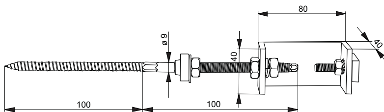
c) Střešní hák nerezový nebo z pozinkované oceli pro vlnité tašky
